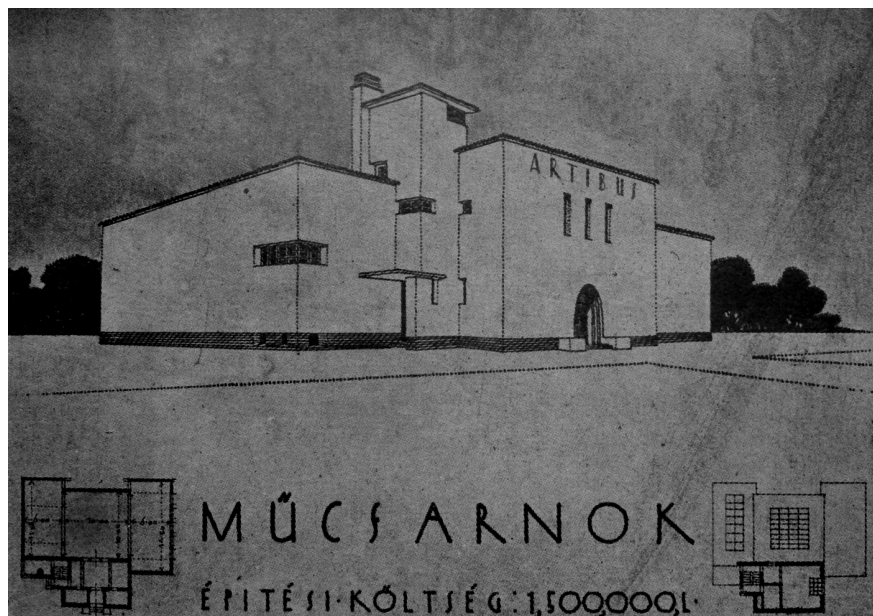
9. Kós Károly: A kolozsvári Műcsarnok terve, 1930.
